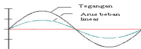
Gambar 1. Karakteristik Gelombang arus beban linier
